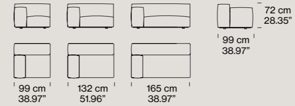
Modulo laterale P 99 cm / Side module D 38.97"
