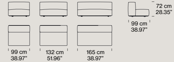
Modulo centrale P 99 cm / Central module D 38.97"
